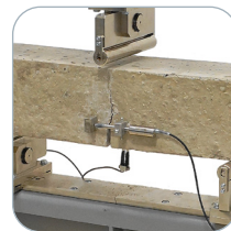
CMOD
