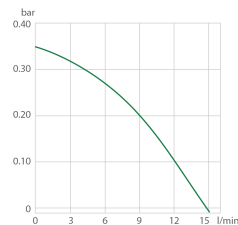
● Pompcapaciteit (Water)
