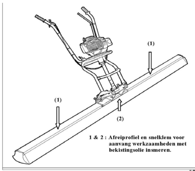
Figuur 9: Afreiprofiel + snelklem met bekistingsolie insmeren
