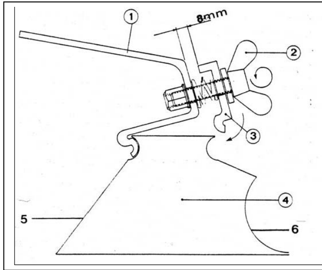
Figuur 6 Snel-aankoppelsysteem.
